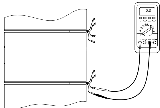
Medición de la corriente mediante un polímetro
