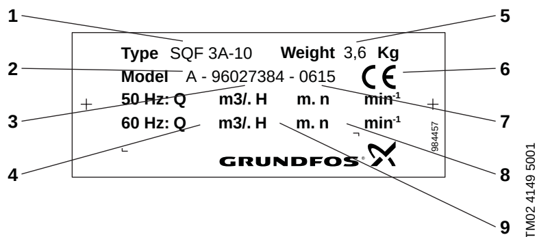
Fig. 2 Placa de características, bombas centrífugas
