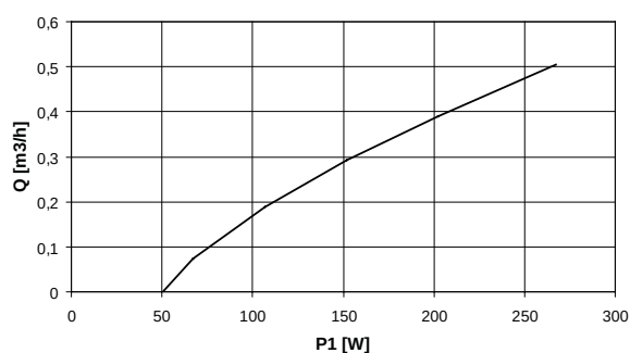
Comprobación de servicio, SQF 1.2 - 2 H = 60 m
