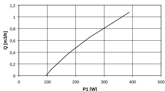
Comprobación de servicio, SQF 3A-10 H = 50 m
