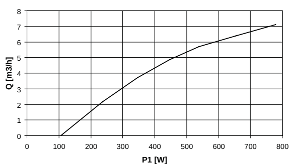
Comprobación de servicio, SQF 8A - 3 H = 10 m
