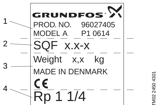
Fig. 1 Placa de características, bomba de rotor helicoidal
