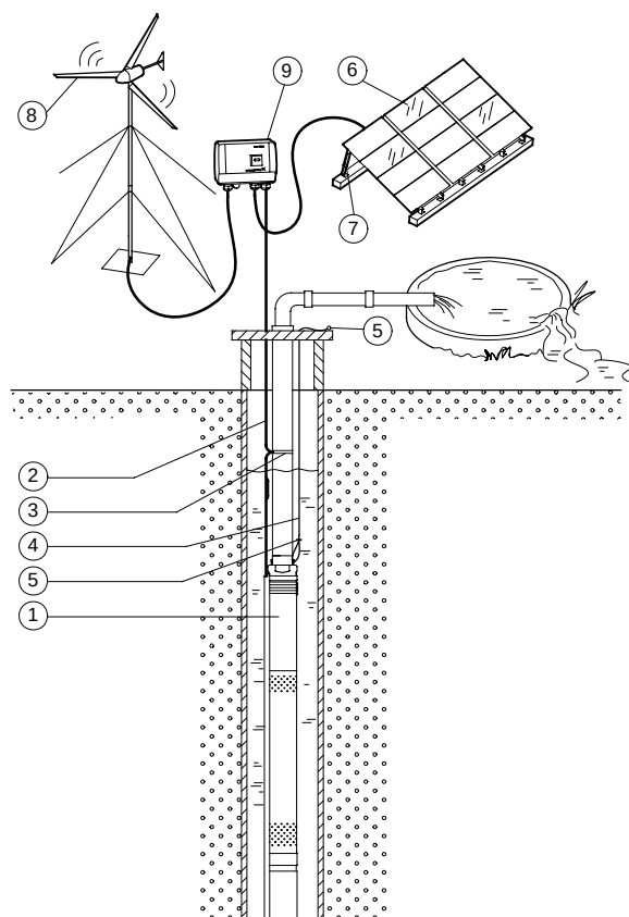
Fig. 17 Principales componentes del sistema combinado
