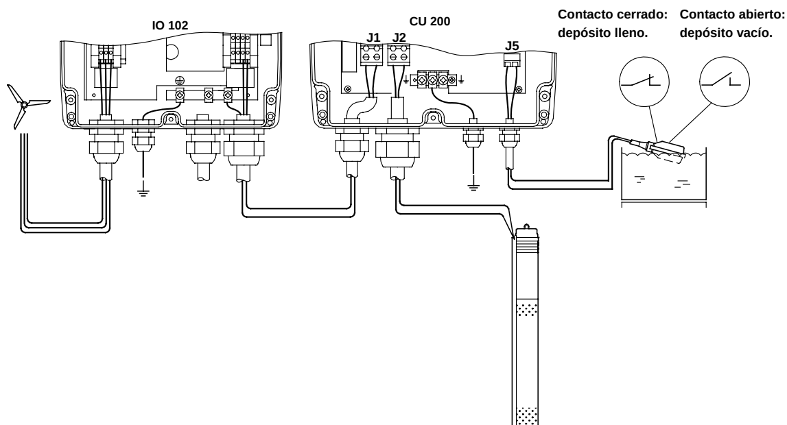
Fig. 16 Cableado interno (y externo) de la caja de control IO 102 y la SQFlex CU 200.
